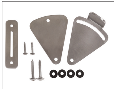
LT-SS-23 • Pestillo para puerta deslizante 3" [76.2 mm] x 2-1/4" [57.3 mm] x 1" [24.5 mm] Acero inoxidable
