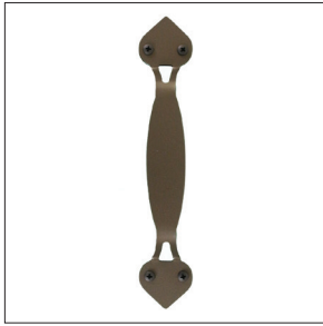
Manija para puerta rodante • 10" [254 mm] x 1-7/8" [45.63 mm] x 1-5/8" [41.28 mm] HD-DSBZ-10 • Bronce pulido (Imagen) HD-DSB-10 • Negro HD-DSSN-10 • Niquelado satinado
